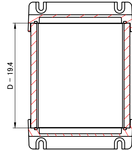
C-C ( 1 : 2.5 )
